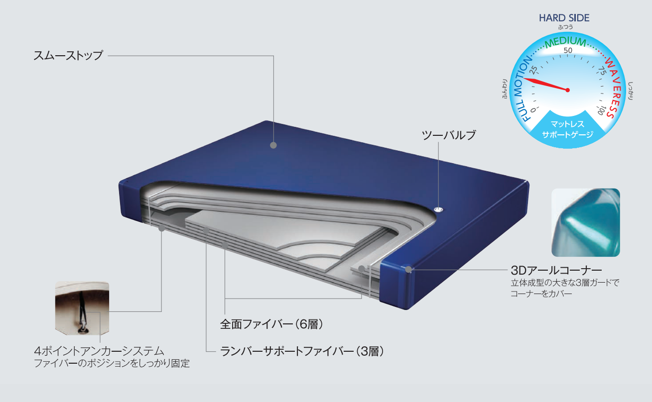
マットレス断面図
